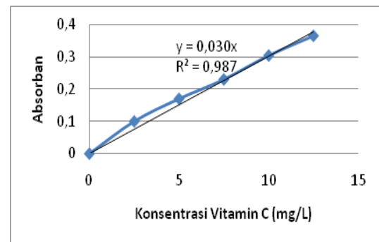
Gambar 2. Kurva hubungan konsentrasi vitamin C (mg/L) dengan absorbansi
