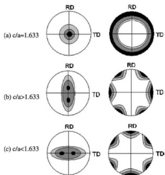
Gambar 1. Simulasi tekstur pengerolan dari (0002) dan (10\bar{1}0) pada logam HCP dengan rasio c/a (a). sama dengan 1,633 (b). lebih besar dari 1,633, and (c). lebih kecil dari 1,633 [10].
