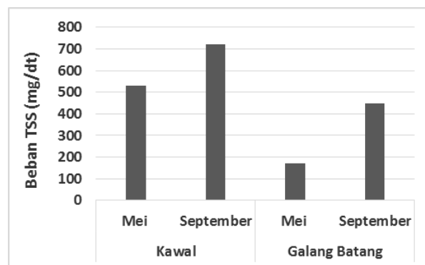
Gambar 3. Beban TSS di muara Sungai Kawal dan Galang Batang pada bulan Mei dan September 2015
