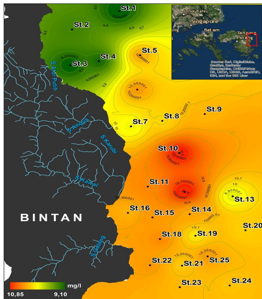
Gambar 6. Sebaran TSS di perairan pesisir Kecamatan Gunung Kijang, Kabupaten Bintang Timur pada bulan September.
