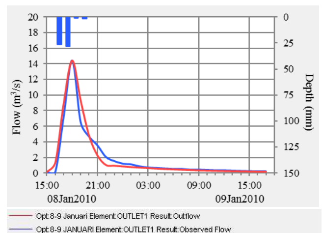
Gambar 6. Hasil Optimalisasi Kalibrasi Hidrograf Banjir Model Tanggal 08-09 Januari 2010
