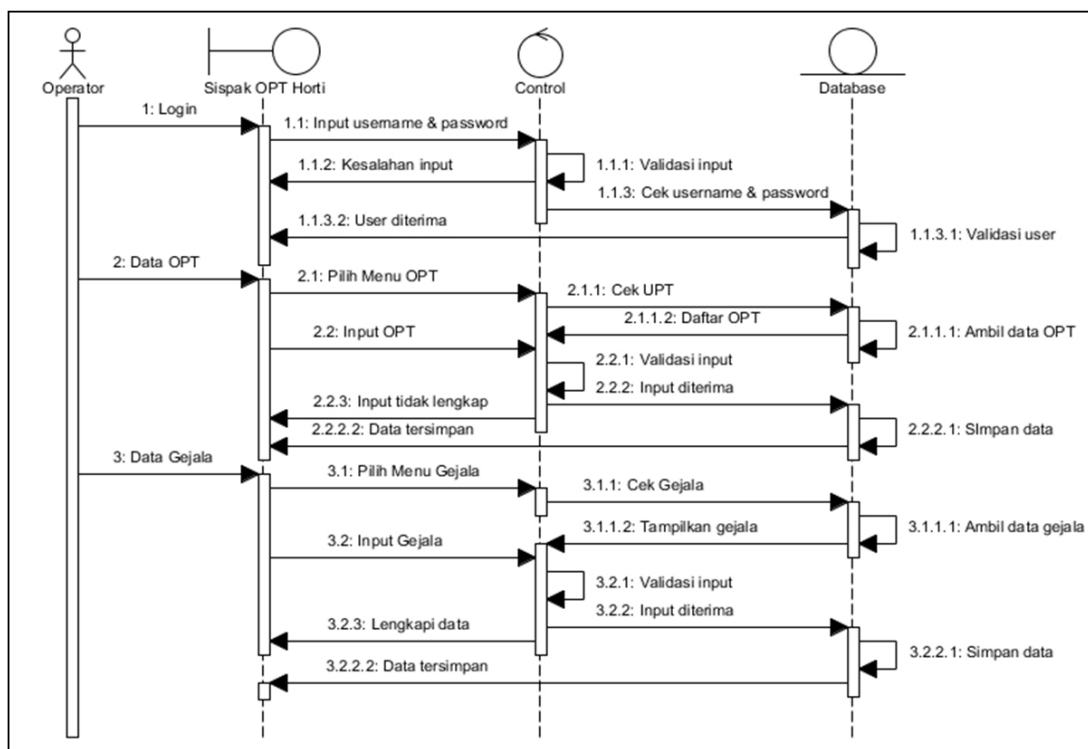
Gambar 10. Diagram sequence pengelolaan OPT
