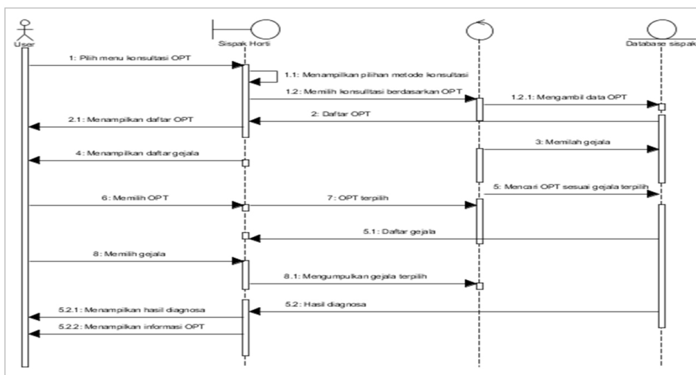
Gambar 9. Diagram sequence konsultasi berdasarkan OPT
