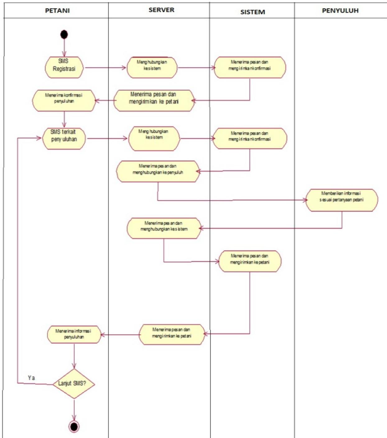
Gambar 2 Activity Diagram Aplikasi Penyuluhan Pertanian
