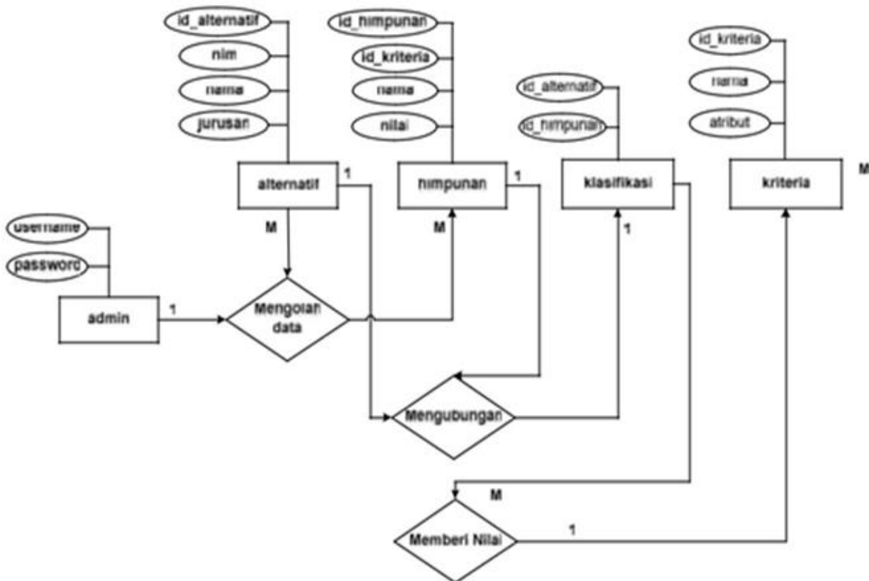
Gambar 13 Relasi Tabel
