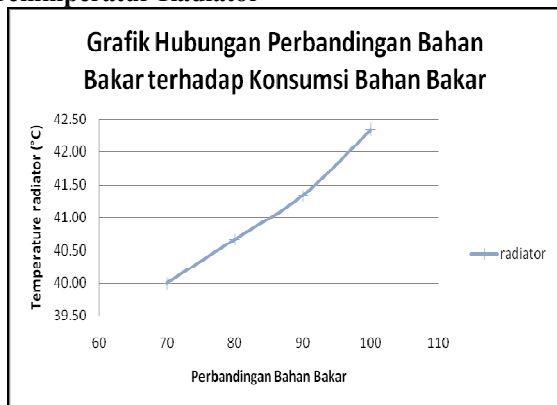
Gambar 9. Grafik hubungan perbandingan bahan bakar terhadap temperatur radiator
