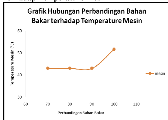
Gambar 8. Grafik hubungan perbandingan bahan bakar terhadap temperature mesin
