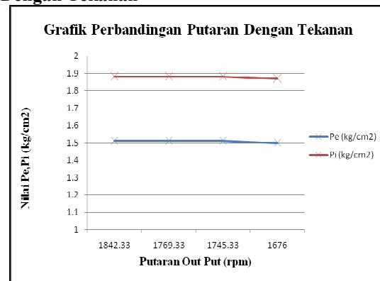
Gambar 4. Grafik Hubungan Perbandingan Antara Putaran Dengan Tekanan
