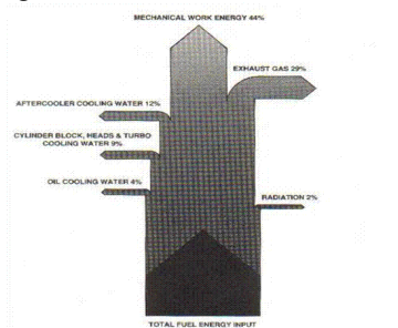
Gambar 1. Bagan konversi energi sebuah mesin diesel
