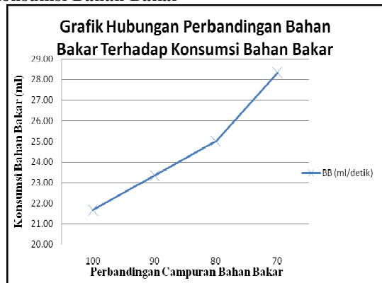
Gambar 6. Grafik Hubungan Perbandingan Bahan Bakar Terhadap Konsumsi Bahan Bakar
