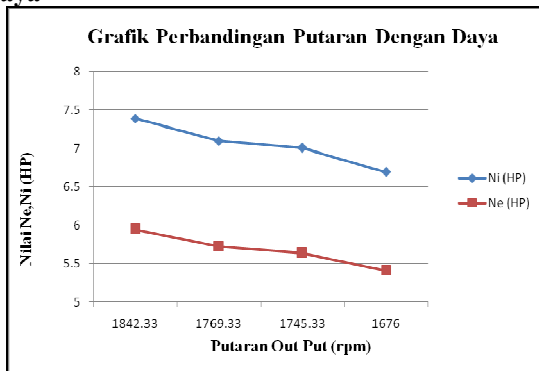
Gambar 5. Grafik hubungan perbandingan antara putaran dengan daya
