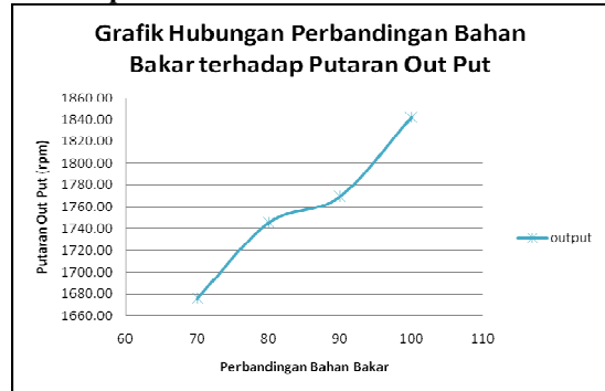
Gambar 7. Grafik hubungan perbandingan bahan bakar terhadap putaran out put
