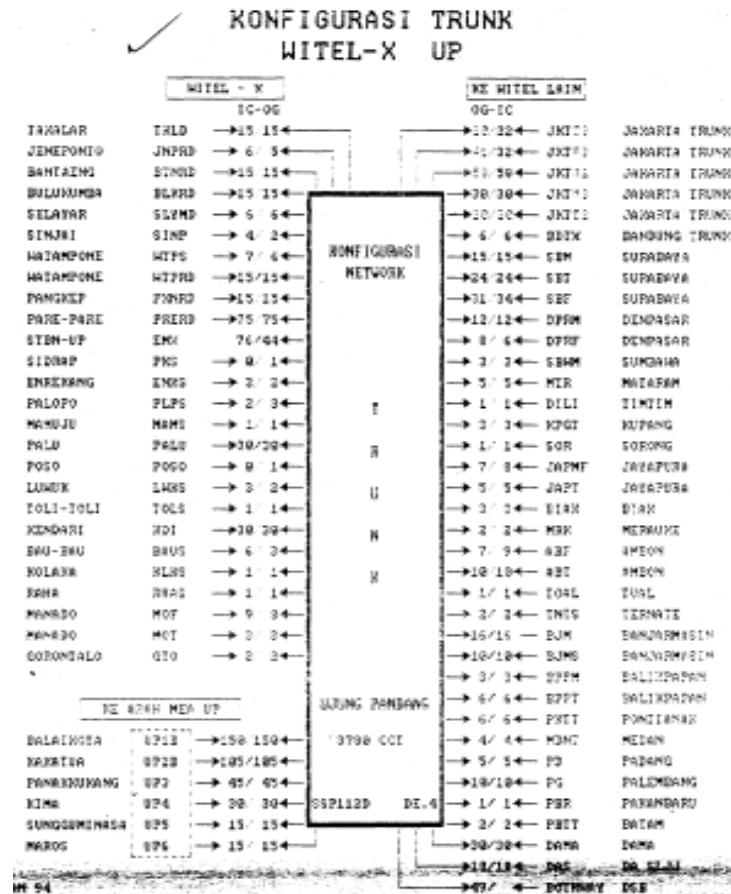
Gambar 8. Konfigurasi trunk WITEL
