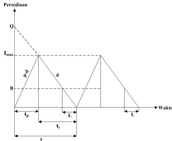
Gambar 2: Grafik EPQ
