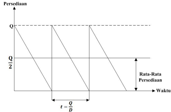
Gambar 1: Grafik EOQ
