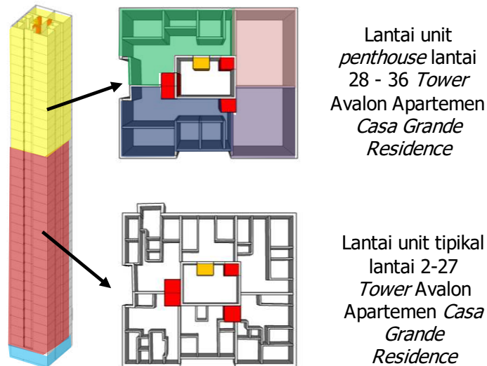
Gambar 7 Analisa Fungsi dengan Fasilitas Unit Berbeda pada Lantai 2 – 27 Tower Avalon Apartemen Casa Grande Residence (Sumber: Marketing Apartemen Casa Grande Residence , 2006, 2015)
