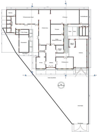
Gambar 2. Denah Baru
