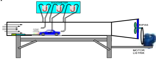
Gambar 5 Wind Tunnel dan Tabung pitot
