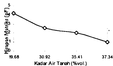
Gambar 2. Kurva hubungan antara hisapan matriks (pF) dengan kadar air tanah di lokasi penelitian
