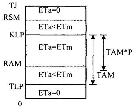
Gambar 1. Hubungan antara nilai ET_a , ET_m dan batas-batas kandungan lengas tanah di perakaran tanaman
