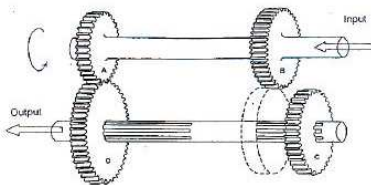
Gambar.7 Posisi gigi 1
