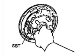
Gambar 16. Melepas Penahan Sepatu Rem
