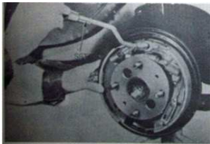
Gambar 15. Melepas pegas pembalik
