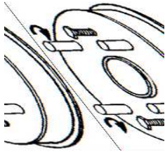
Gambar 14. Melepas Tromol Rem
