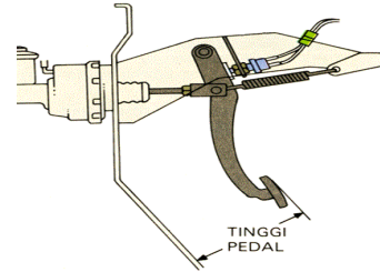
Gambar 12. Pemeriksaan Tinggi Pedal
