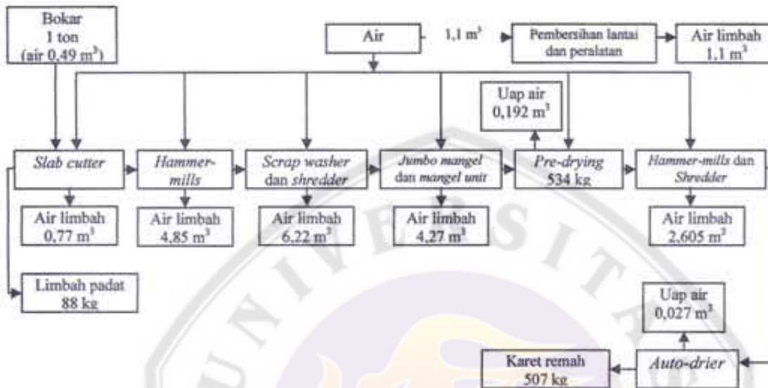
Gambar 4. Air proses untuk pengolahan bokar menjadi karet remah
