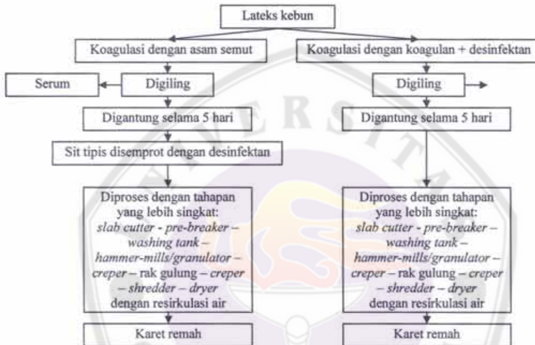
Gambar 6 Rancang bangun industri karet remah berbasis karet rakyat berdasarkan konsep produksi bersih
