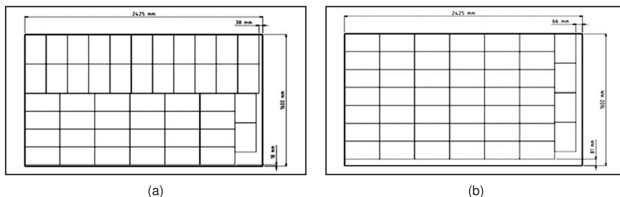
Gambar 2. Pola penyusunan kemasan pada bak pick-up (a) 48 kemasan, (b) 46 kemasan.
