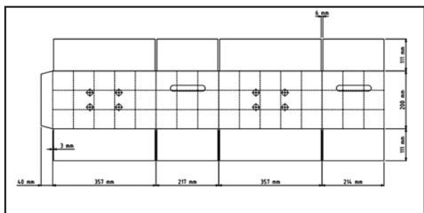
Gambar 3. Desain kemasan hasil rancangan partisi.
