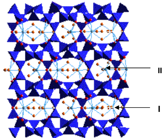
Gambar 4. Kerangka struktur Sangkar Zeolit Clinoptilolite (Bayah dan Lampung) dalam ruang 3D hasil program Crystal Maker , S10R (I), diameter Poros = 10,685 Å dan S8R (II) diameter PorosI = 8,193 Å
