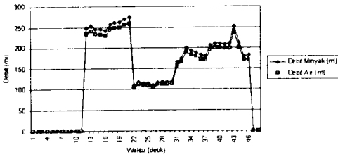
Gambar3. Perbandingan Debit Minyak dan Air Pada Perbandingan 30:70, Suhu 85°C Ulangan II
