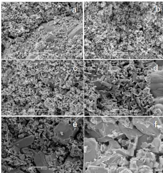
Gambar 3. Hasil SEM pada perbesaran 5000X untuk (a) sampel A 1s , (b) sampel B 1s , (c) sampel A 2s , (d) sampel B 2s , (e) sampel A 3s dan (f) sampel B 3s .
