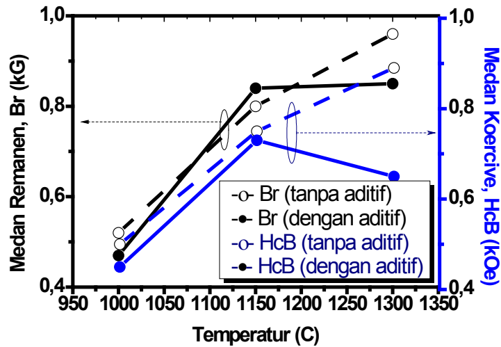
Gambar 4. Kurva medan magnetik remanen ( B_r ) dan medan magnetik coercive ( H_{cB} ) terhadap temperatur sintering tanpa aditif (o) dan dengan aditif (●).
