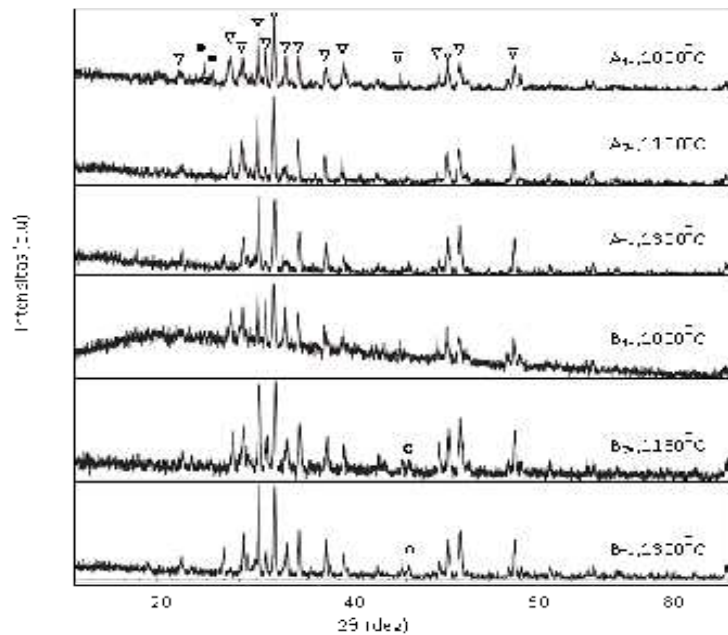
Gambar 2. Pola XRD \text{BaFe}_{12}\text{O}_{19} untuk (a) sampel A_{1s} , (b) sampel A_{2s} , (c) sampel A_{3s} , (d) sampel B_{1s} , (e) sampel B_{2s} , (f) sampel B_{3s} . ( \nabla adalah puncak \text{BaFe}_{12}\text{O}_{19} , \bullet adalah puncak impuritas dari \text{BaCO}_3 dan \text{Fe}_2\text{O}_3 yang belum bereaksi sempurna, dan o adalah puncak impuritas yang diperkirakan dari puncak senyawa \text{CuO-TiO}_2 ).
