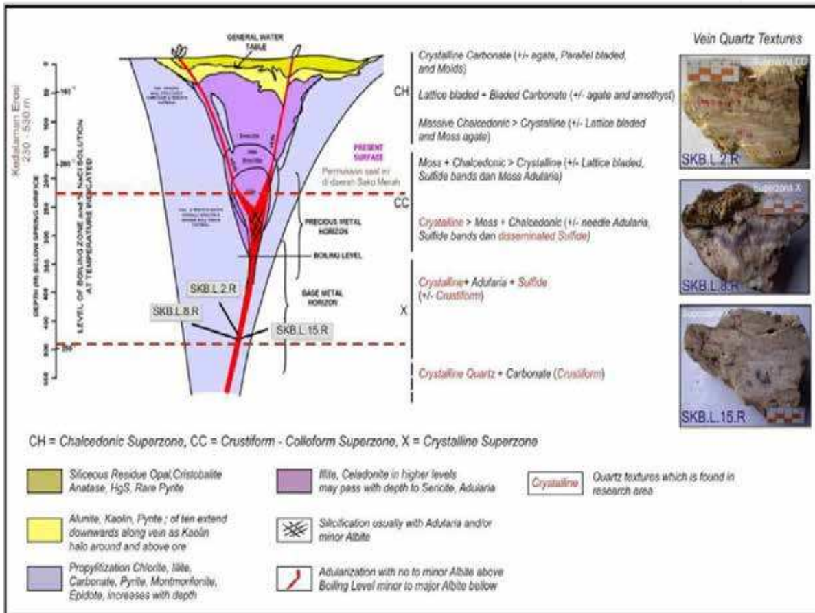
Gambar 6. Model zonasi tekstur vein kuarsa dan hubungannya dengan distribusi kadar emas-perak (Au-Ag) dalam sistem mineralisasi vein epitermal di daerah penelitian
