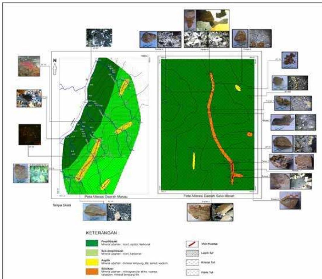
Gambar 3. Peta alterasi dan mineralisasi daerah Manau dan Sako Merah
