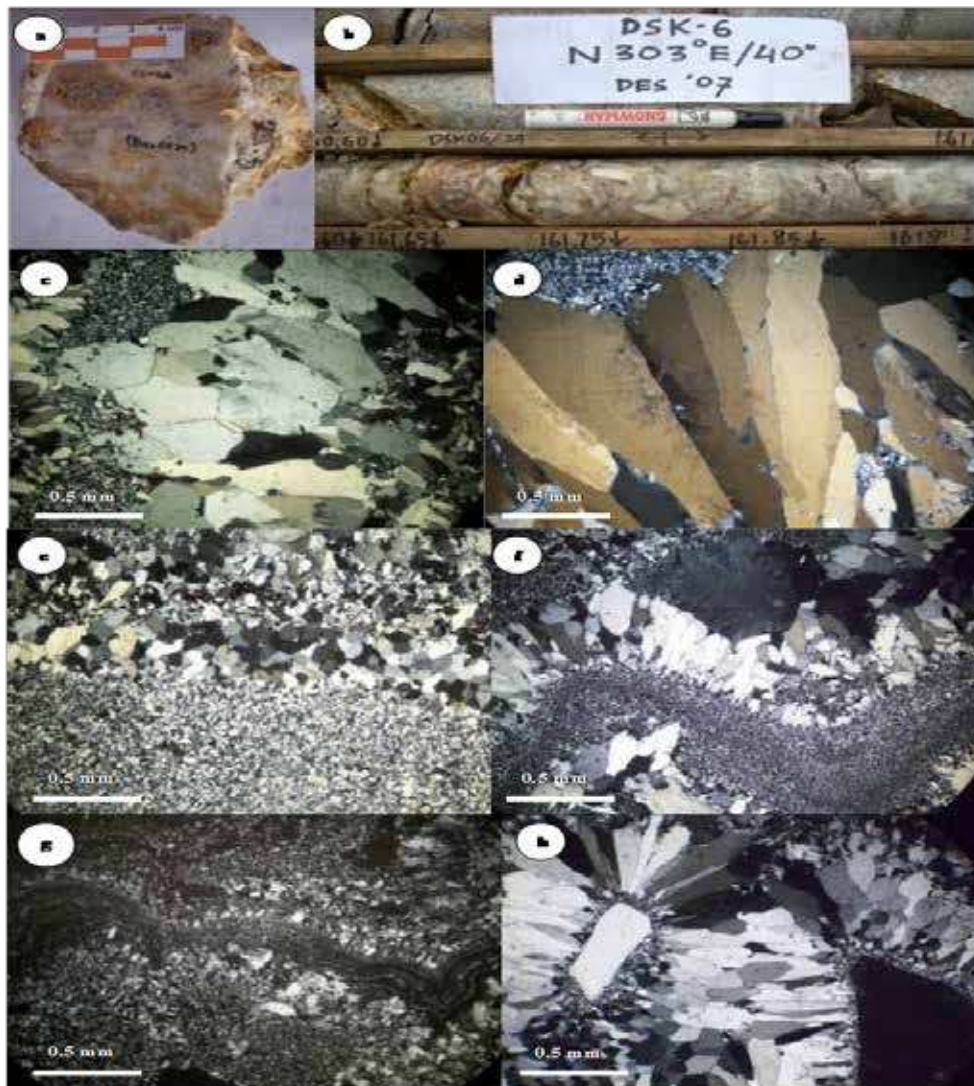
Gambar 4 (a) Contoh urat kuarsa breksia pada Bukaan 3; (b) Urat kuarsa pada DSK 6; (c) Sayatan tipis urat kuarsa bertekstur comb ; (d) Urat kuarsa bertekstur zonal; (e) Sayatan tipis urat kuarsa bertekstur saccharoidal ; (f) Sayatan tipis urat kuarsa bertekstur colloform berasosiasi chalcidonic ; (g) Sayatan tipis urat kuarsa bertekstur crustiform banding ; (h) Sayatan tipis urat kuarsa bertekstur comb .
