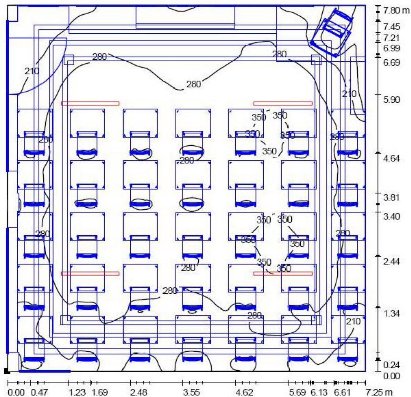
Gambar 6. Model layout penyebaran cahaya pada ruang kelas XI IPS 2
