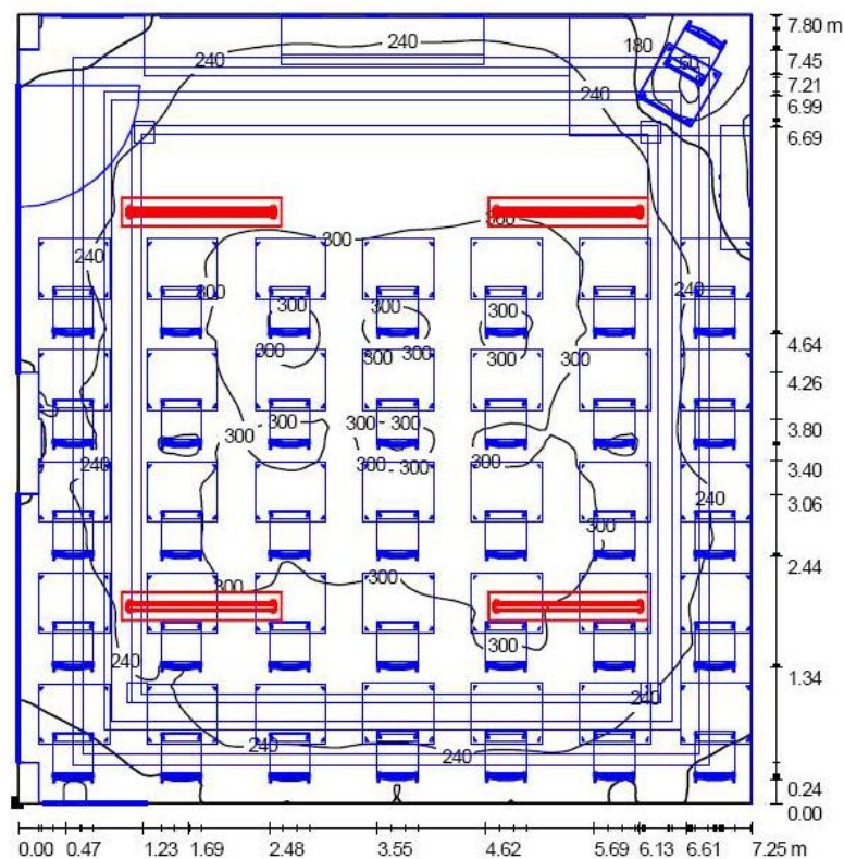
Gambar 9. Model layout penyebaran cahaya pada ruang kelas XII IPS 2
