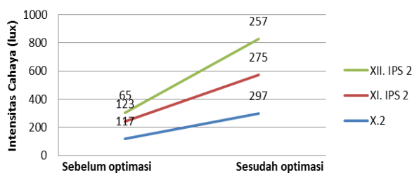
Gambar 12. Grafik hasil optimasi ruang kelas XI IPS 2
