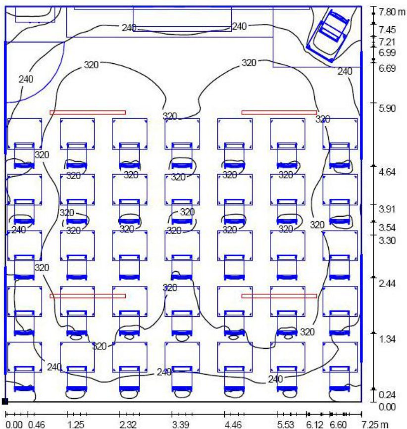
Gambar 3. Model layout penyebaran cahaya pada ruang kelas X2
