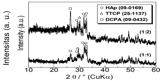
Gambar 4. Pengaruh molar rasio TTCP dan DCPA terhadap pola difraksi sinar X hydroxyapatite pada perendaman selama 5 hari
