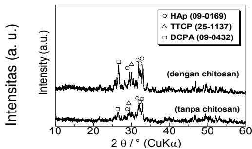
Gambar 7. Pengaruh penambahan chitosan terhadap pola difraksi sinar X hydroxyapatite pada perendaman selama 1 hari dengan menggunakan molar rasio TTCP dan DCPA 1:1
