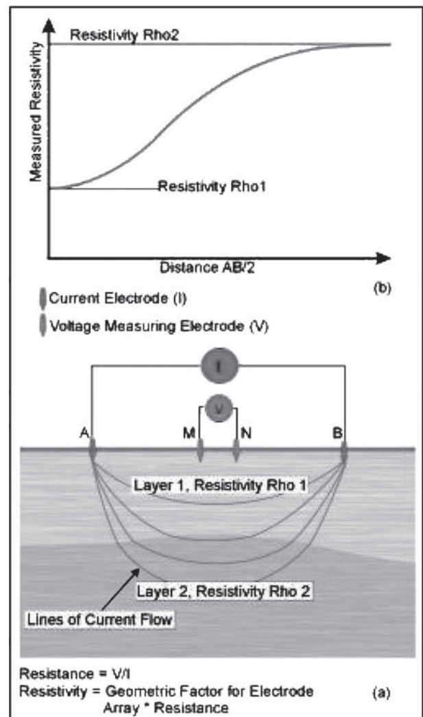
Gambar 4. Konfigurasi Elektroda Metoda Resistivity
