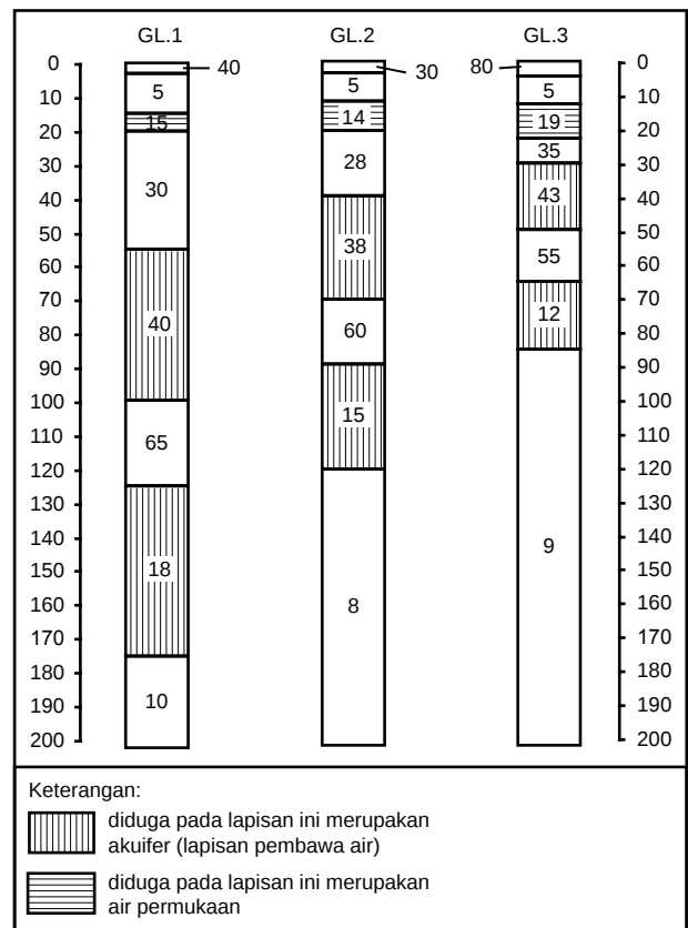
Gambar 6. Penampang Tegak Tahanan Jenis di Kantor KLH, By Pass Jakarta Timur
