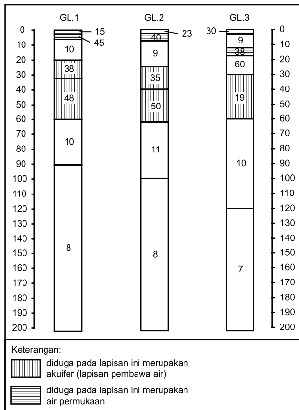
Gambar 5. Penampang Tegak Tahanan Jenis di Perum Taman Duta, Cimanggis Depok.
