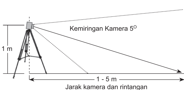
Gambar 1. Ilustrasi pengambilan citra pemandangan di depan traktor
