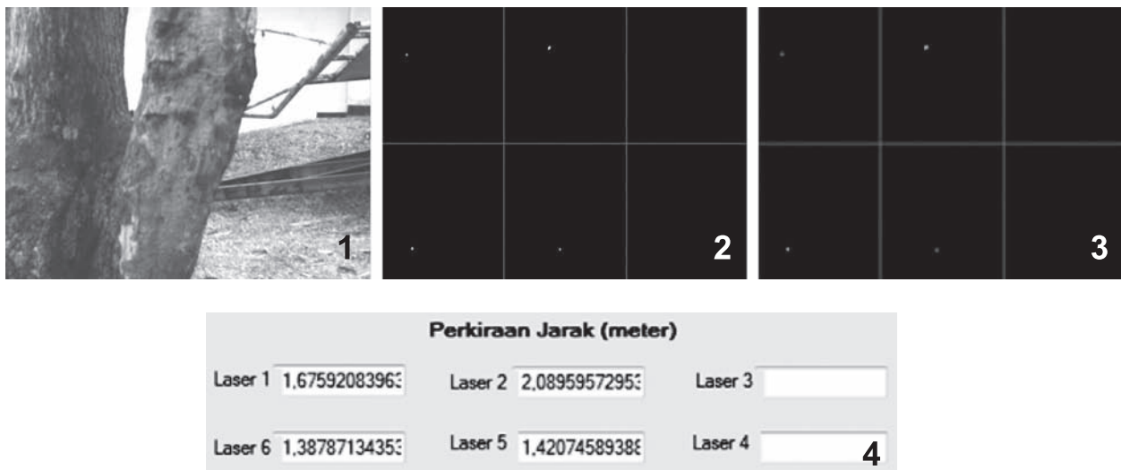
Gambar 6. Urutan operasi yang dikenakan untuk mendeteksi jarak rintangan pada citra dengan rintangan 1 m di depan: 1) citra yang diambil, 2) setelah dilakukan operasi thresholding , 3) setelah dilakukan operasi opening dan 4) informasi perkiraan jarak
