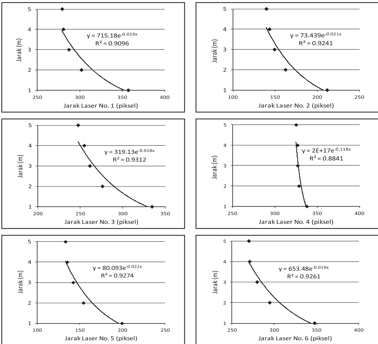
Gambar 4. Hubungan jarak laser No. 1 hingga No. 6 terhadap pusat citra dengan jarak rintangan pada pengambilan citra untuk kalibrasi
