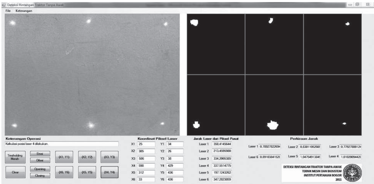
Gambar 3. Tampilan program pada saat proses thresholding merah terhadap citra dinding dengan jarak 1 m
