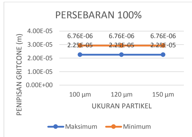
Gambar 22 Penipisan yang terjadi pada persebaran 100%
