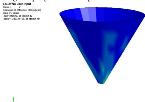
Gambar 5 Von Mises Pada Gritcone untuk spesimen 1
