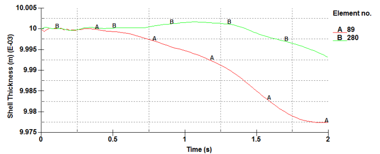
Gambar 13 Pengaruh Waktu terhadap Ketebalan pada Gritcone
