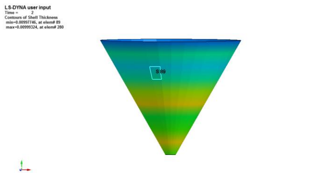
Gambar 12 Ketebalan Gritcne pada persebaran Material 100%, pada ukuran partikel 100 µm
