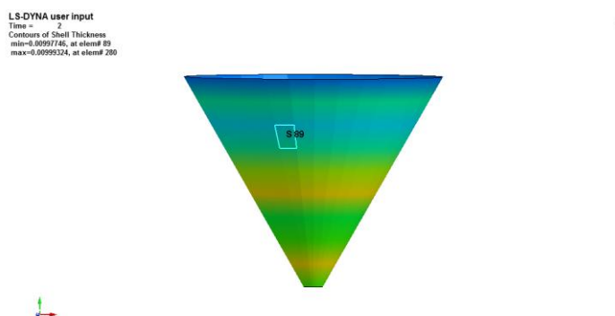
Gambar 18 Ketebalan Gritcone pada persebaran Material 100%, pada ukuran partikel 150 µm
