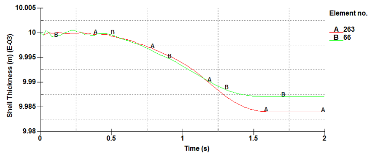
Gambar 7 Pengaruh Waktu terhadap Ketebalan pada Gritcone
