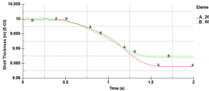
Gambar 10 Pengaruh Waktu terhadap Ketebalan pada Gritcone
