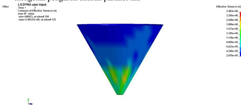
Gambar 20 Von Misses Pada Gritcone untuk spesimen 6
