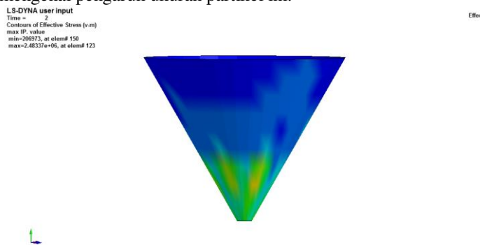
Gambar 17 Von Misses Pada Gritcone untuk spesimen 5
