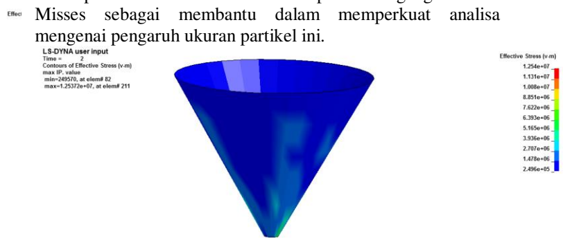
Gambar 8 Von Mises Pada Gritcone untuk spesimen 2
