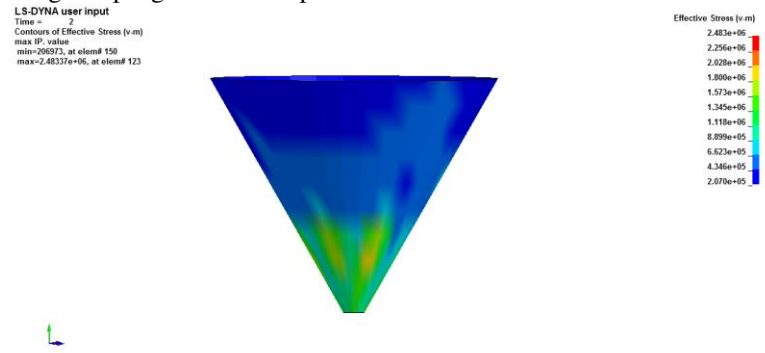
Gambar 14 Von Misses Pada Gritcone untuk spesimen 4
