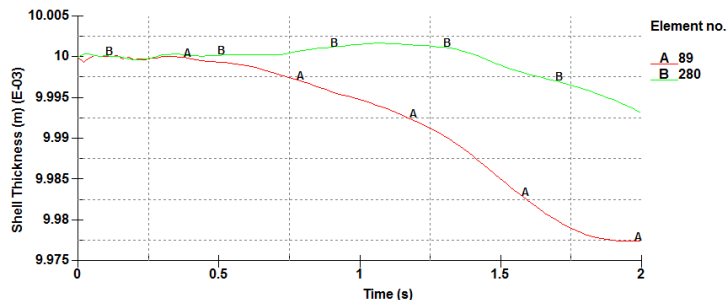
Gambar 19 Pengaruh Waktu terhadap Ketebalan pada Gritcone
