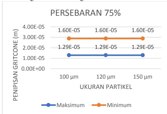
Gambar 21 Penipisan yang terjadi pada persebaran 75%
