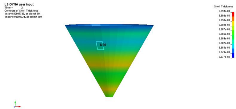
Gambar 15 Ketebalan Gritcne pada persebaran Material 100%, pada ukuran partikel 120 µm
