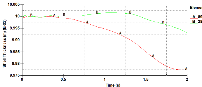
Gambar 16 Pengaruh Waktu terhadap Ketebalan pada Gritcone
