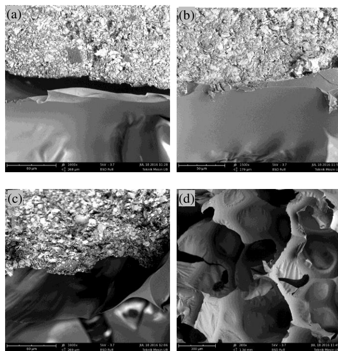
Gambar 3. SEM coating permukaan melintang a) BaM/Pani Jaumann layer 1000x (b) BaM/PPy Jaumann layer 1500x (c) BaM/PET Jaumann layer 1000x (d) Pu foam
