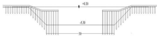
Gambar 8. Potongan Memanjang Krib Beton pada Sta. 800
