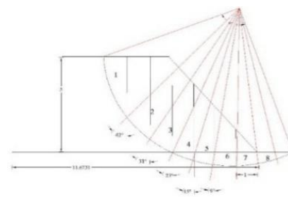
Gambar 9. Irisan Bidang Longsor
