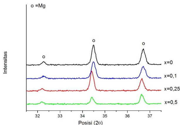
Gambar 2. Pola difraksi sinar-x untuk sudut pendek 2\theta = 31,5-37,5 setelah mechanical milling untuk komposisi penambahan aluminium
