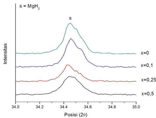
Gambar 6. Pola difraksi sinar-x untuk sudut pendek 34°-35° setelah proses hidriding untuk serbuk Mg_{2-x}Al_xNi ( x=0;0,1;0,25;0,5 ) dengan heat treatment 385°C.
