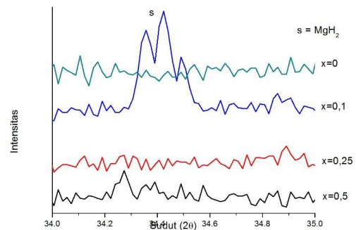
Gambar 10. Pola difraksi sinar-x untuk sudut pendek 34°-35° setelah proses hidriding setelah annealing serbuk Mg_{2-x}Al_xNi ( x=0;0,1;0,25;0,5 ) pada serbuk heat treatment 385°C.
