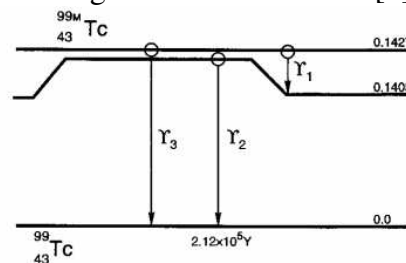
Gambar 1. Skema peluruhan Tc^{99m} dengan waktu paro 6,02 jam [4].
