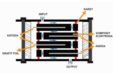
Gambar 3 Prototip desalinasi FTC
