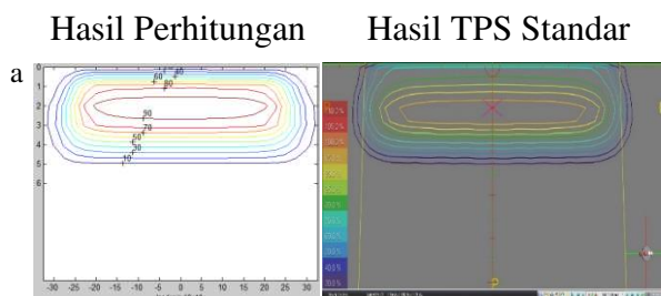
Gambar 7. Bentuk kurva isodosis pada beberapa luas lapangan yang dihasilkan oleh perhitungan dan TPS standar, a. Luas Lapangan 10 x 10 cm 2 b. Luas Lapangan 15 x 15 cm 2 c. Luas Lapangan 20 x 20 cm 2 d. Luas Lapangan 25 x 25 cm 2
