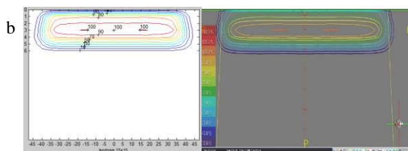
Gambar 7. Bentuk kurva isodosis pada beberapa luas lapangan yang dihasilkan oleh perhitungan dan TPS standar, a. Luas Lapangan 10 x 10 cm 2 b. Luas Lapangan 15 x 15 cm 2 c. Luas Lapangan 20 x 20 cm 2 d. Luas Lapangan 25 x 25 cm 2
