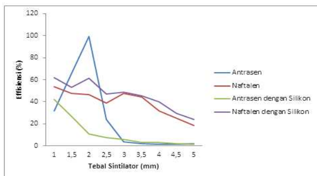
Gambar 8. Grafik efisiensi sintilator
