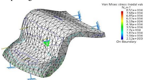
Gambar 7. Distribusi Tegangan pada Konsep Existing
