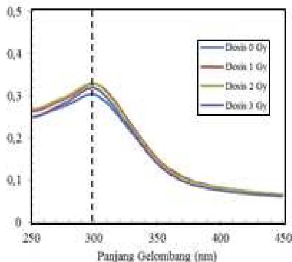
Gambar 4 Spektrum absorbansi UV larutan nanopartikel CeO 2 untuk berbagai dosis radiasi gamma untuk nanopartikel CeO 2 dikalsinasi pada temperatur 400 °C
