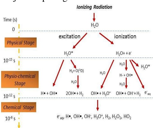
Gambar 2. Skema Peristiwa Radiolisis [11] Nanopartikel Cerium Dioksida
