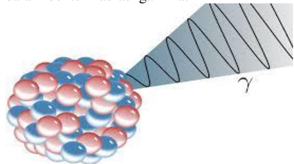
Gambar 1. Peluruhan Sinar Gamma
