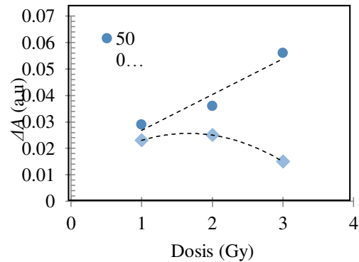
Gambar 6 Nilai \Delta A larutan nanopartikel CeO 2 untuk berbagai dosis radiasi gamma
