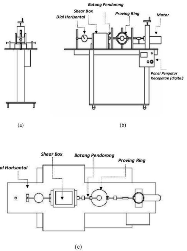
Gambar 3. Alat uji Geser Modifikasi (Rusdiansyah,2015) [4]
