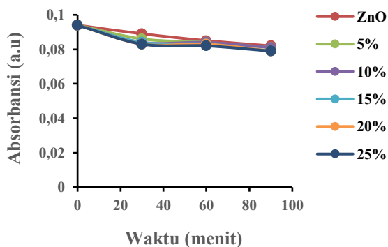
Gambar 5. Fotokatalitik degradasi zat warna Direct Blue 71
