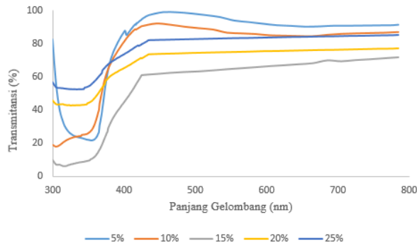
Gambar 2. Transmittansi UV-Vis lapisan tipis ZnO:Co dengan variasi doping Co
