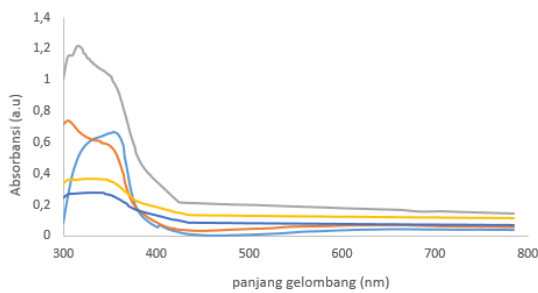
Gambar 3. Absorbansi UV-Vis lapisan tipis ZnO:Co dengan variasi doping Co
