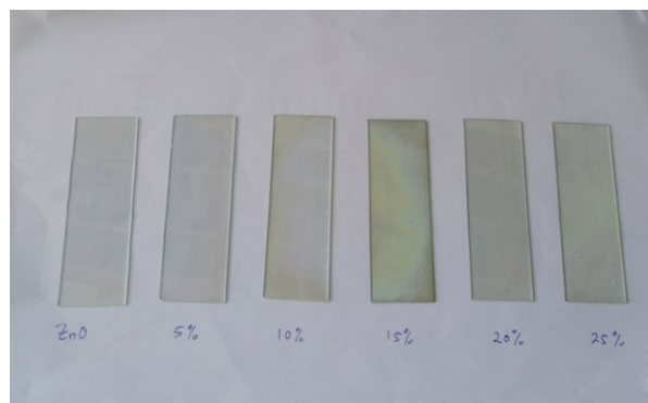
Gambar 1. Lapisan tipis ZnO:Co yang dideposisi pada substrat kaca dengan variasi doping Co 5%, 10%, 15%, 20% dan 25%
