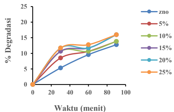
Gambar 6. Efisiensi fotokatalitik lapisan tipis ZnO:Co
