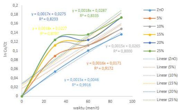
Gambar 7. Kinetik fotodegradasi dengan variasi konsentrasi Co
