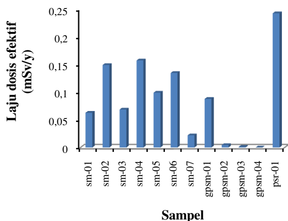
Gambar 9. Laju dosis efektif sampel semen (sm), gypsum (gpsm) dan pasir (psr)
