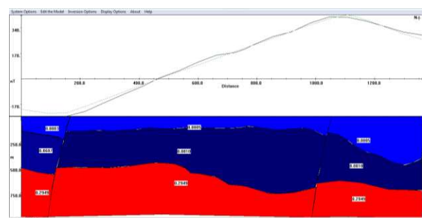
Gambar 12. Hasil Pemodelan sayatan B-B'
