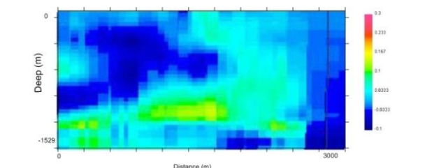
Gambar 16. Sayatan A-A' dalam pemodelan 3D
