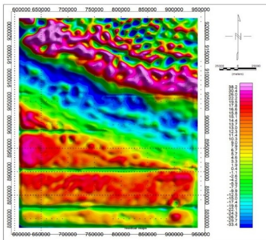
Gambar 4 Kontur anomali residual
