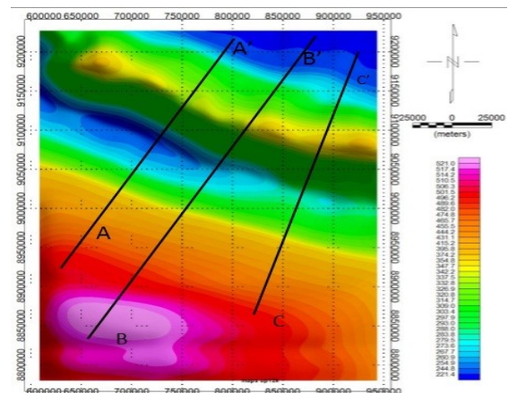
Gambar 5 Peta anomali regional dengan 3 lintasan
