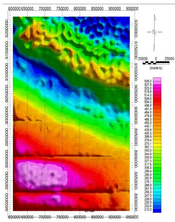
Gambar 2 Kontur anomali hasil proyeksi bidang datar
