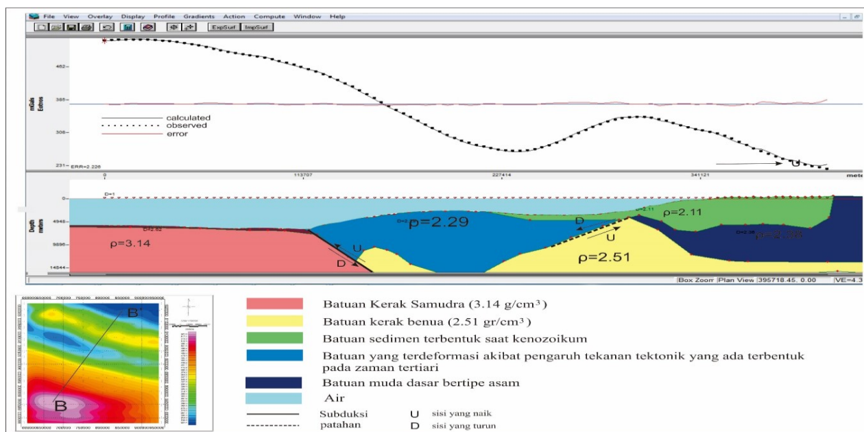
Gambar 6 Pemodelan struktur bawah permukaan pada lintasan-2
