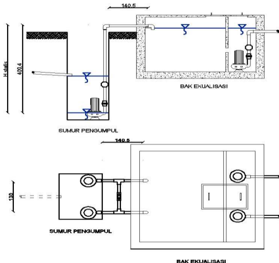
Gambar 3. Skema pemompaan dari bak ekualisasi
