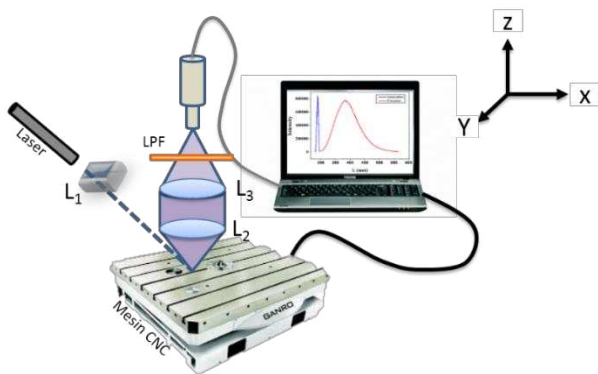
Gambar 2. Rangkaian alat optik
