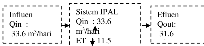
Gambar 6. Kestimbangan massa air
