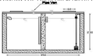
Gambar 9. Potongan bak ekualisasi
