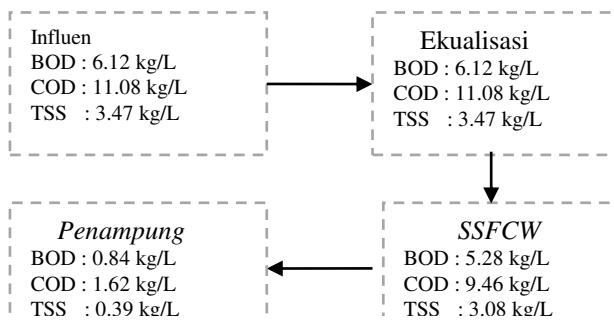
Gambar 5. Massa balance polutan dalam sistem IPAL
