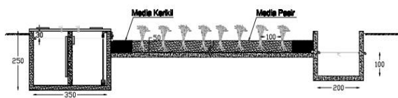
Gambar 11. Potongan SSFCW
