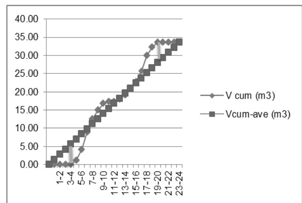
Gambar 7. Volume Kumulatif bak ekualisasi
