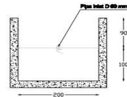
Gambar 13. Potongan Kolam Penampung
