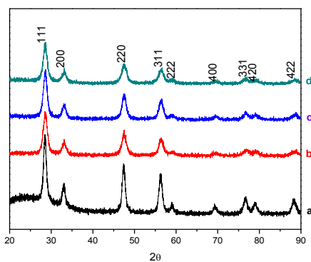
Gambar 3. Spektra difraksi sinar-x nanopartikel \text{CeO}_2 dengan berbagai persentase Zn (a) 0%, (b) 5%, (c) 10%, (d) 20%
