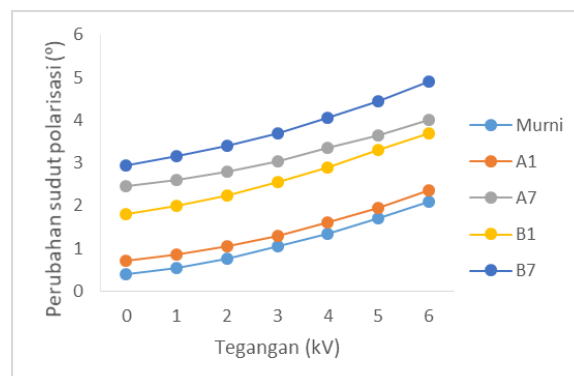
Gambar 2 Perubahan sudut polarisasi transmisi elektrooptis.
