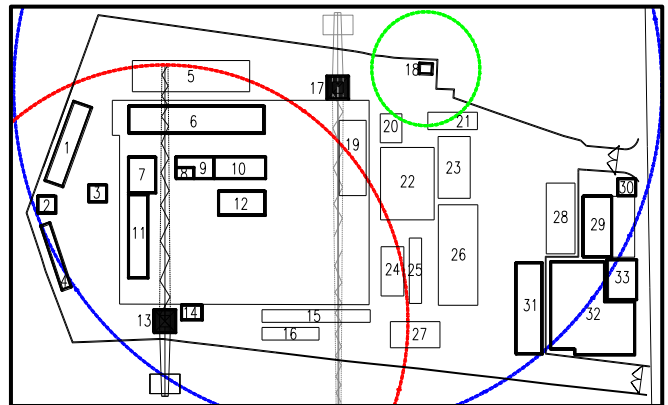
Gambar. 4. Eksisting site layout (skenario 0)
