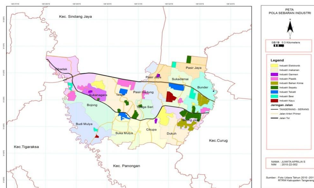
Gambar 7. Peta Analisis Pola Sebaran Industri
