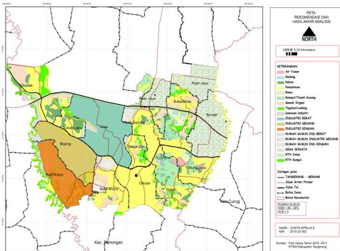
Gambar 8 Rekomendasi Spasial pola sebaran industri
