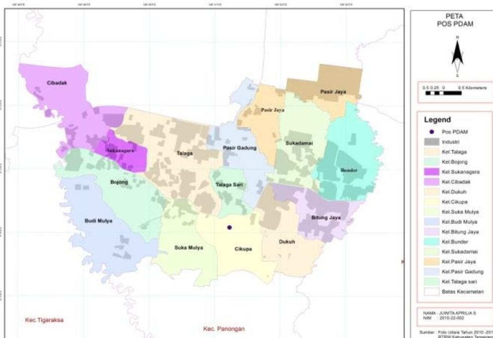
Gambar 5. Peta Analisis Hidrologi
