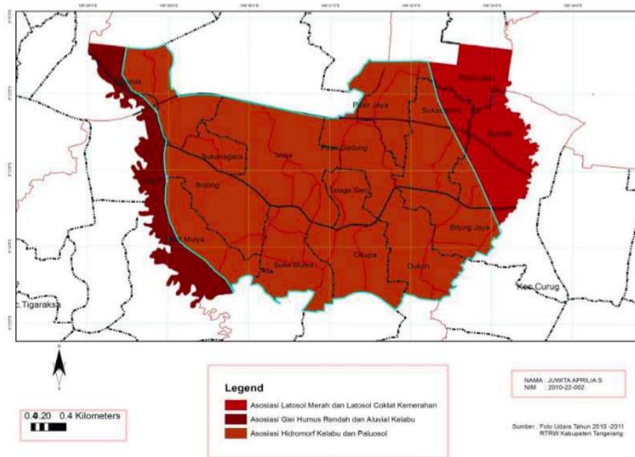
Gambar 3 Peta Analisis Geologi
