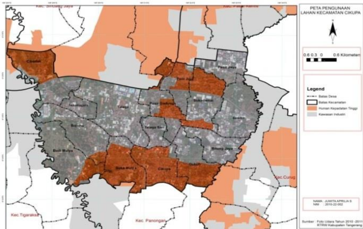
Gambar 2. Analisis Penggunaan Lahan
