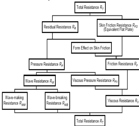
Gambar 3. Diagram Komponen Koefisien Hambatan Total Kapal [6]
