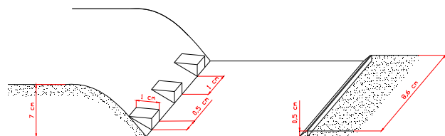
Gambar 2. Dimensi kolam olakan Model 1
