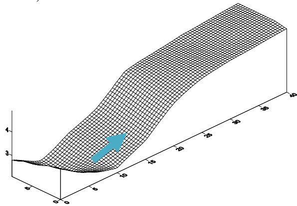
Gambar 16. Pola gerusan dihilir bendung dengan debit 2,097 \times 10^{-3} \text{ m}^3/\text{det}
