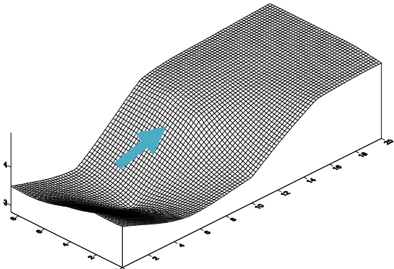
Gambar 12. Pola gerusan dihilir bendung dengan debit 1,297 \times 10^{-3} \text{ m}^3/\text{det}
